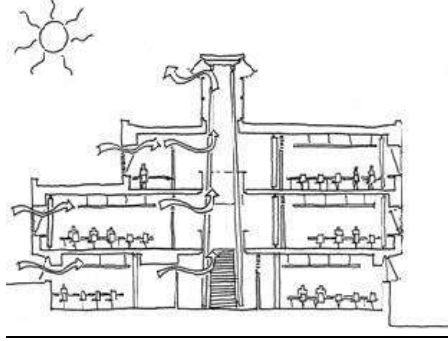
شكل (4) مقطع رأسي يظهر حركة الرياح وملقف الهواء
